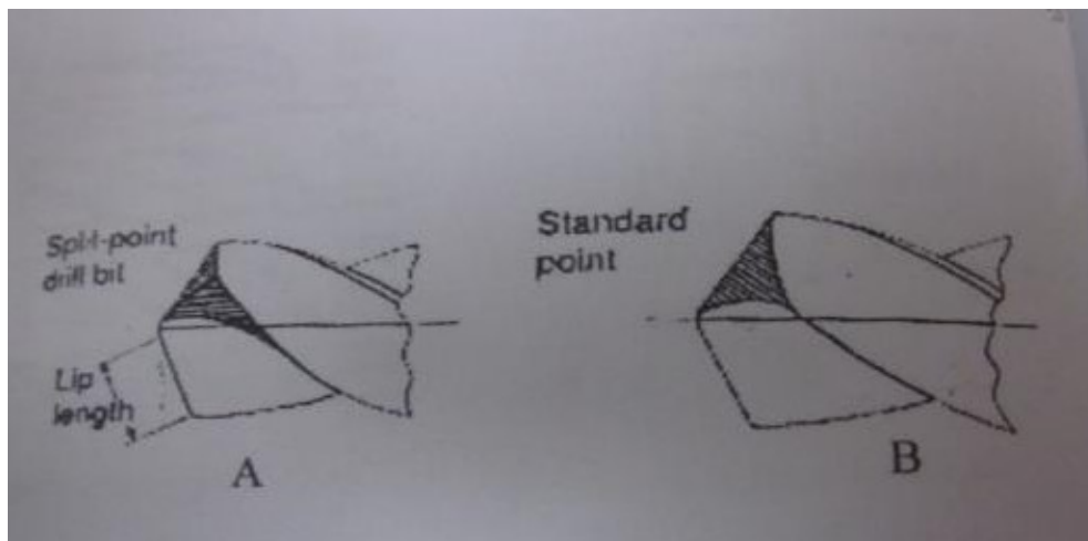
شکل ۵. تفاوت لبه پرنده سرمته split point (A) و سرمته استاندارد (B).
