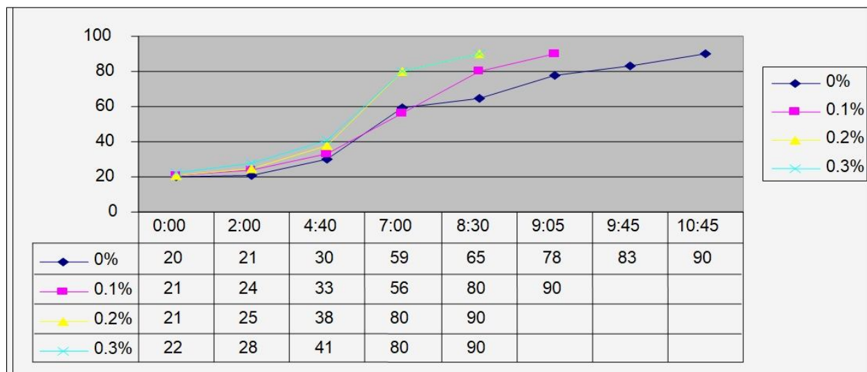
نمودار ۴. اسیدیته بر حسب درجه دورنیک در ماست پروبیوتیکی بیفیدوباکتریوم بیفیدوم طی گرماخانه گذاری.
