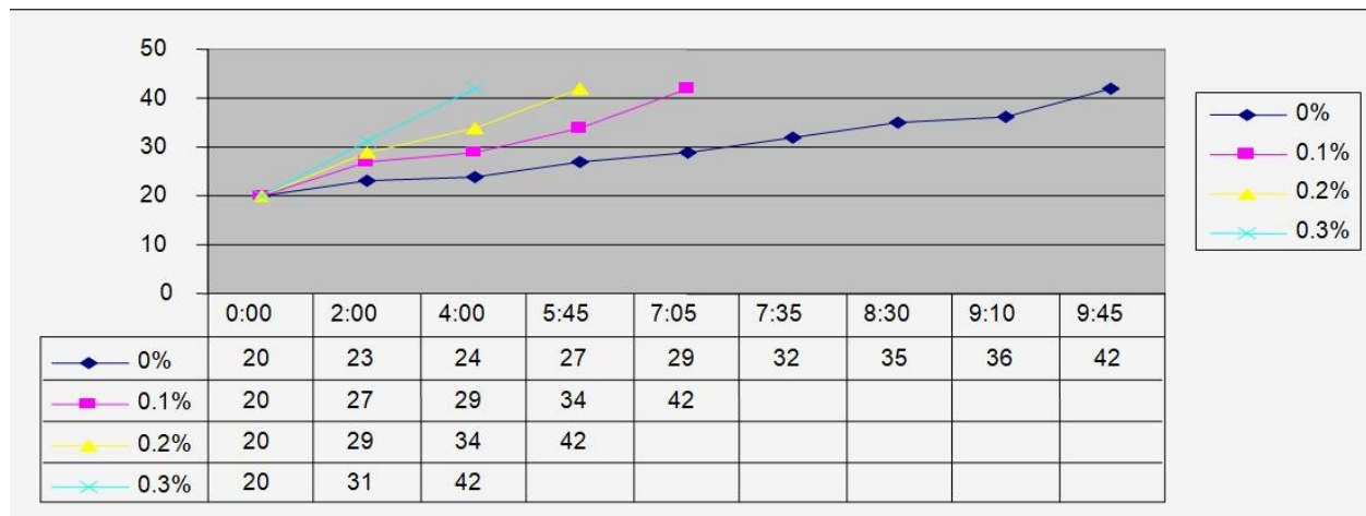
نمودار ۱. اسیدیته بر حسب درجه دورنیک در شیر لاکتوباسیلوس اسیدوفیلوس طی گرمخانه گذاری.
