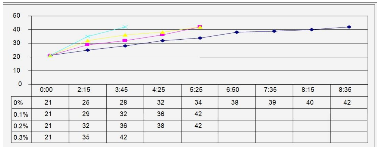
نمودار ۳. ارزیابی اسیدیته بر حسب درجه دورنیک در شیر پروبیوتیکی بیفیلوباکتریوم بیفیدوم طی گرمخانه گذاری.
