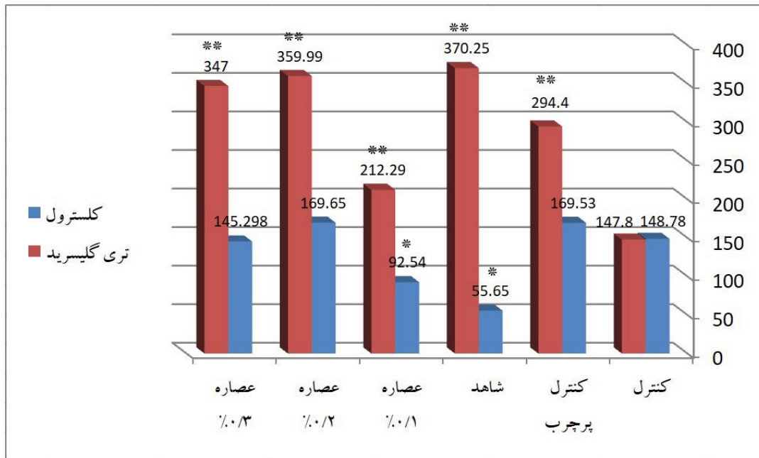
نمودار ۵. مقایسه تأثیر شیر پروبیوتیکی لاکتوباسیلوس اسیدوفیلوس بر میزان کلسترول و تری گلیسرید سرمی (mg/dL) موشهای صحرایی. * مقایسه میانگین و انحراف معیار میزان کلسترول با گروه کنترل. ** مقایسه میانگین و انحراف معیار میزان تری گلیسرید با گروه کنترل.
